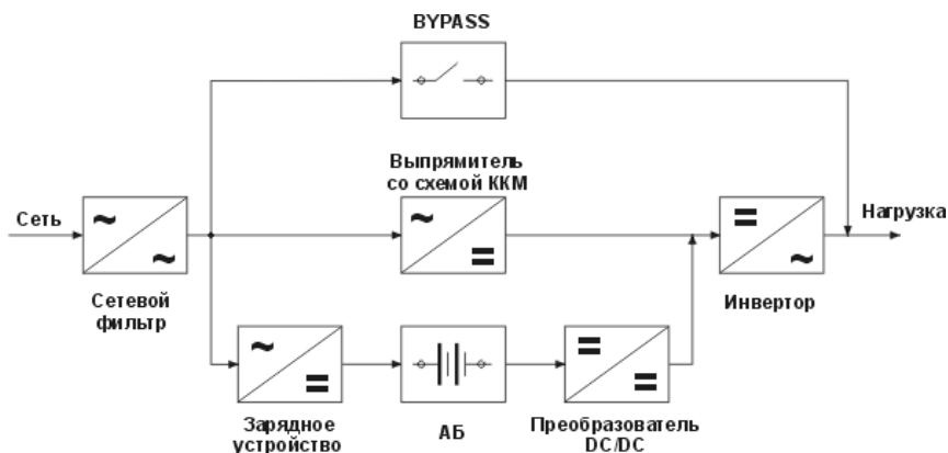
Рис. 2 Структурная схема ИБП
